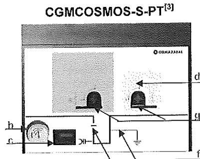
Фигура 1.9: Синоптична схема на шкаф CGMCOSMOS-S-PT [3]
